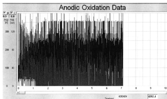
그림 2. A graphic of anodizing oxidation at impulse voltage 350 V, pulse cycle 10 mS
