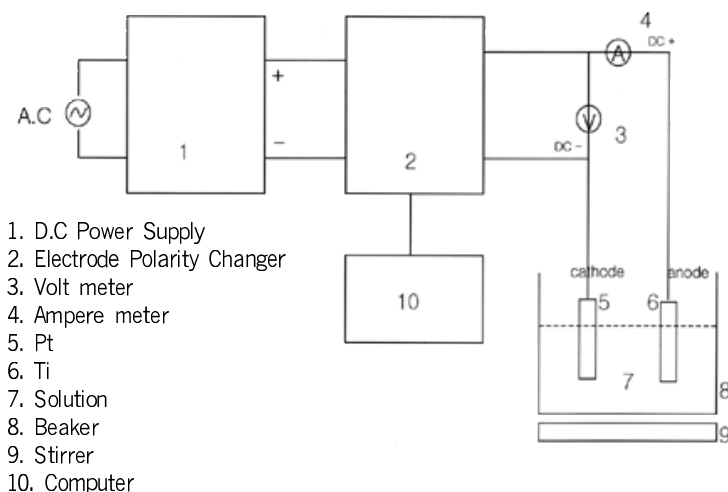
그림 1. Schematic illustration of the anodizing apparatus.
