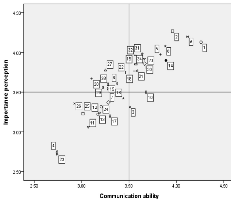
Fig. 1. IPA analysis
